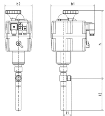
2) Aufbauzubehör Temperaturableitung
