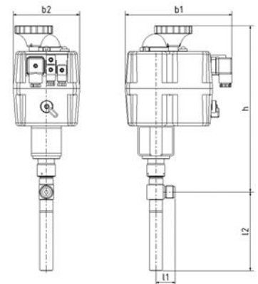
2) Aufbauszubehör Temperaturableitung
